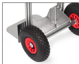
Wielbevestiging geschroefde wielbevestiging, eenvoudige bandenwissel.
