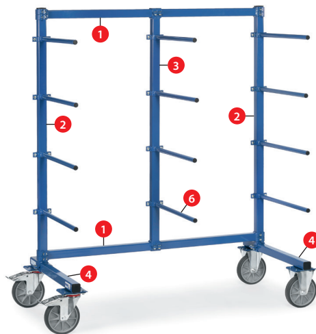
Onderdelen voor Draagarmwagen
